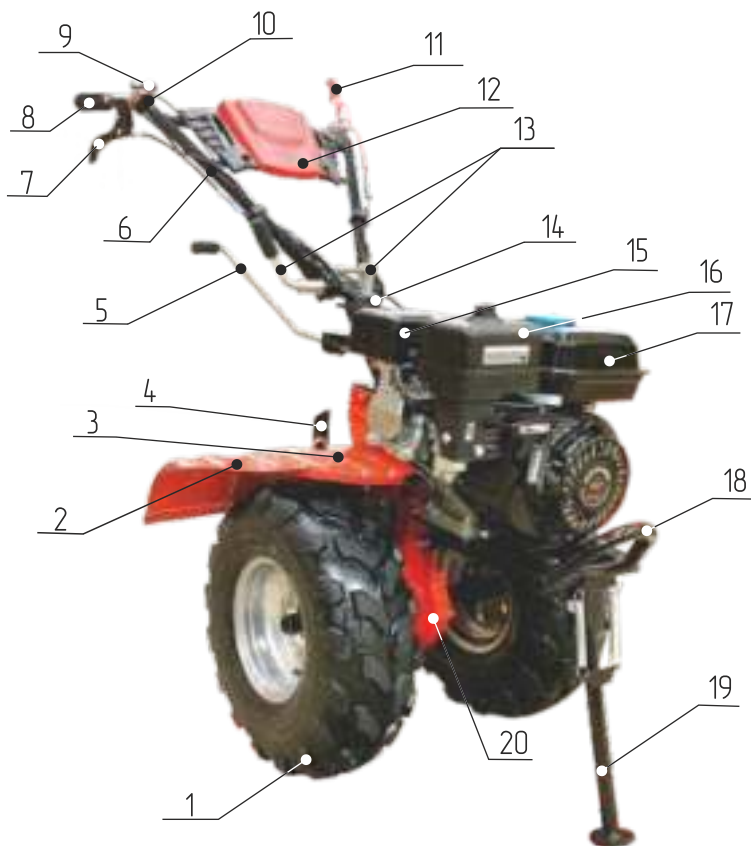
Рис.1 Мотоблок (общий вид)
